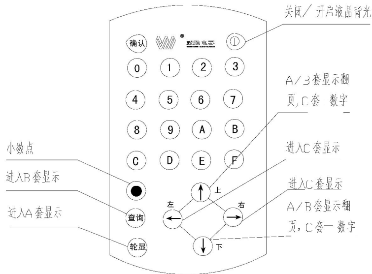
遥控器外形图
