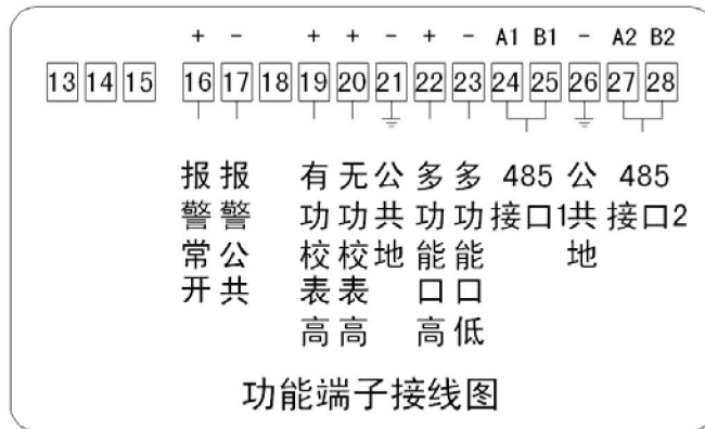
内置继电器电能表辅助端子排列图
