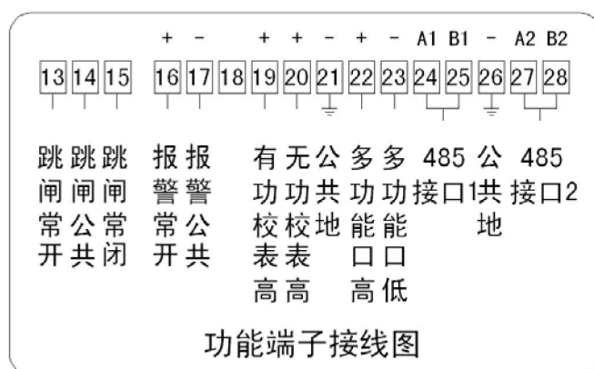
外置继电器电能表辅助端子排列图
